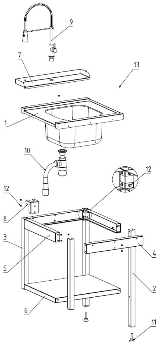
Рисунок 1- Схема сборки изделия (правая загрузка кассет)
