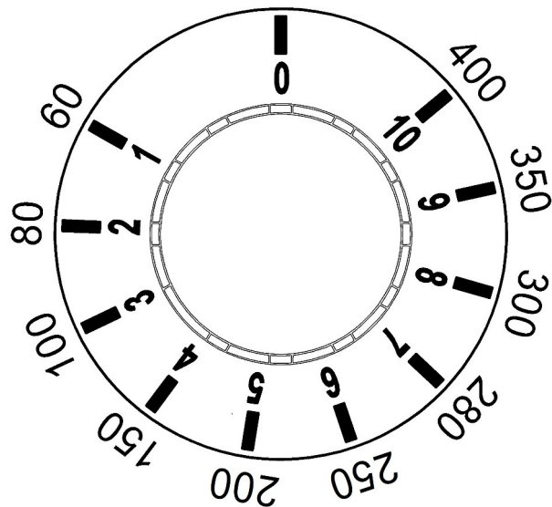
Рис.3 Соответствие числовым отметкам шкалы значениям температуры.
