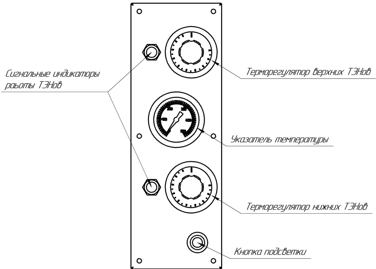
Рис.2 Общий вид панели управления.
