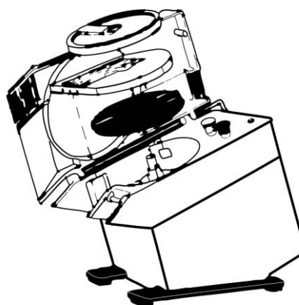
Положение диска (2)
